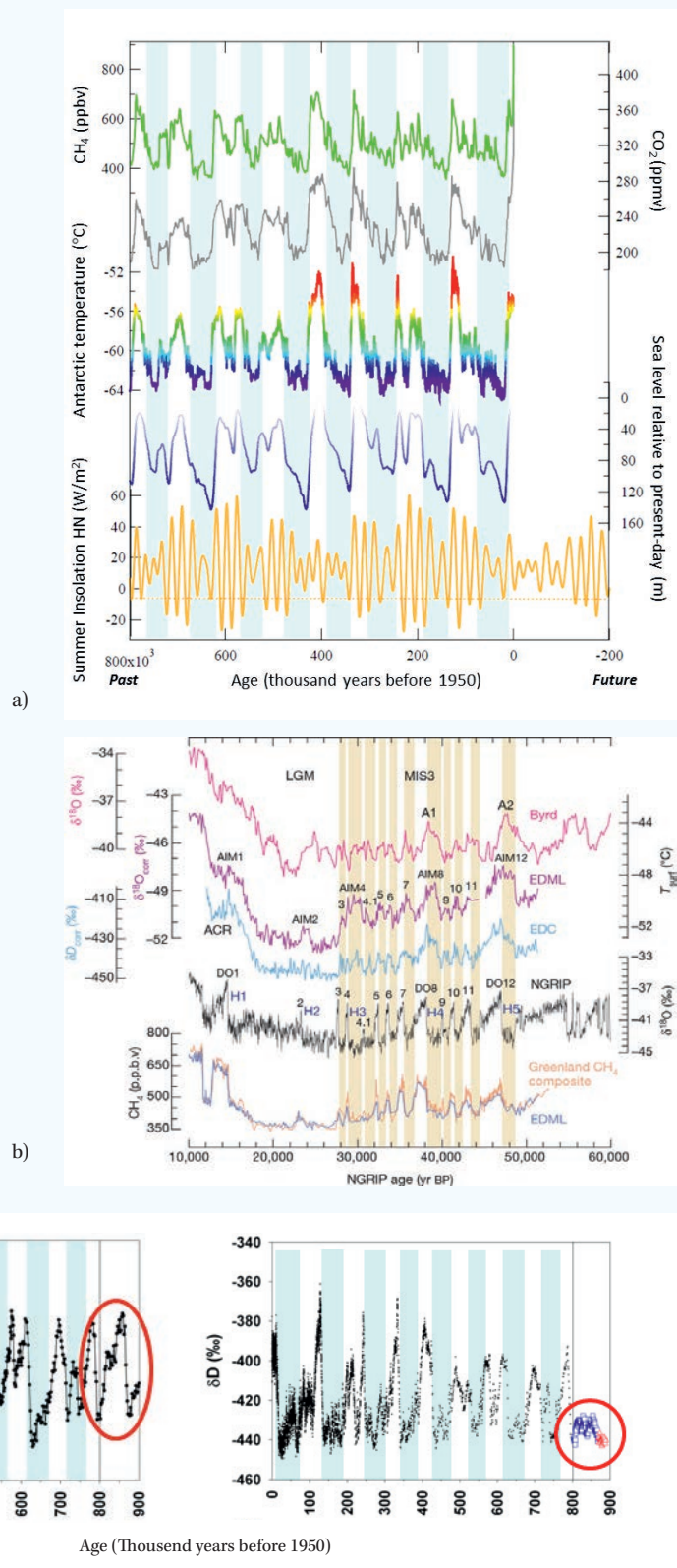
Figure 1 : Données paléoclimatiques du projet EPICA : a) 8 cycles climatiques naturels (époques glaciaires en bleu clair) : températures, gaz à effet de serre, niveau marin (Masson-Delmotte et al., 2010) ; b) synchronisation HN (NGRIP)/HS (EDC, EDML) au cours du dernier glaciaire (EPICA Community, 2006) et c) discordance entre proxys de température dans les sédiments marins (benthic \delta^{18}O , bas) et dans la glace basale (haut et milieu : \delta D_{glace} ) d'EPICA (Tison et al., 2015).
