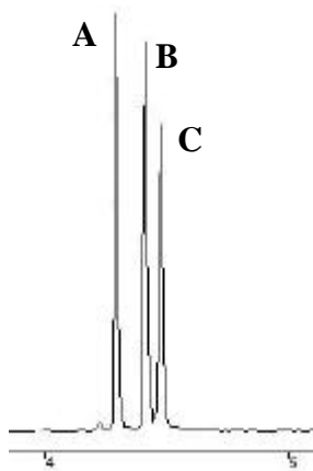
Fig. 1 : PeCDD/Fs (min)
