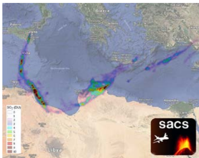
Fig. 6 : Pluim van zwaveldioxide (SO 2 ) die op 26 december 2018 uit de vulkaan Etna in Zuid-Italië is uitgestoten. De kaart toont de verspreiding van de pluim onder de werking van de wind in de lagere atmosfeer. Deze gegevens worden gebruikt als indicator voor de aanwezigheid van vulkaanas als onderdeel van de Aviation Control Support Service (ACSS) die op het BIRA is ontwikkeld om informatie te verstrekken over vulkanische gevaren. © BIRA-IASB/ESA/DLR
