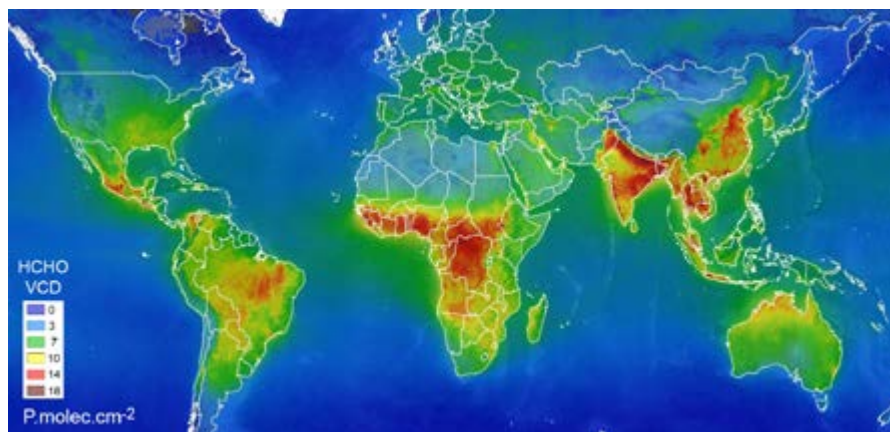
Fig. 5 : Kaart van troposferische kolommen van formaldehyde ( \text{HCHO} ) die de gemiddelde jaarlijkse verspreiding van bronnen van vluchtige organische stoffen (VOS) over de wereld laat zien. Deze emissies zijn ofwel van natuurlijke oorsprong die verband houden met de vegetatiecycli, ofwel veroorzaakt door bosbranden, voornamelijk in tropische gebieden, ofwel door antropogene vervuiling (met name in China). © BIRA-IASB/ESA/DLR
